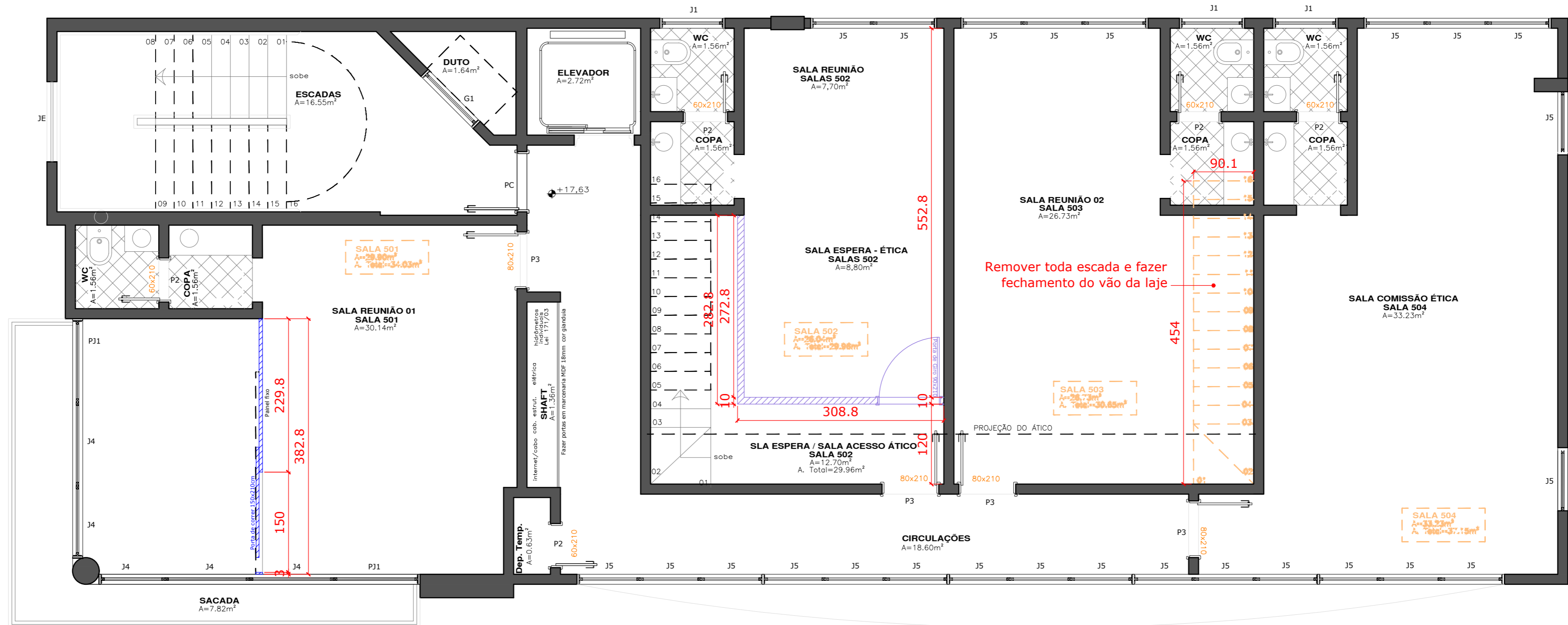
PLANTA MODIFICAÇÃO DE OBRA - QUINTO PAVIMENTO Escala 1/50
