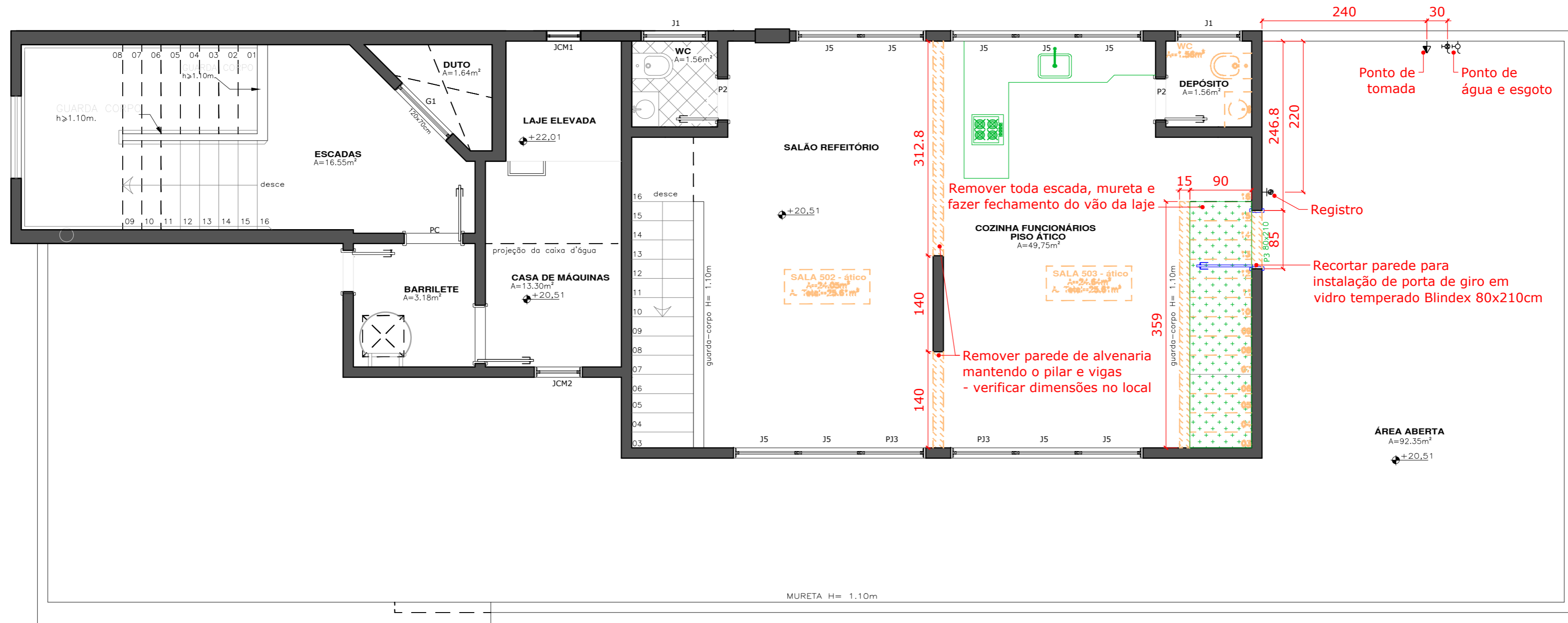
PLANTA MODIFICAÇÃO DE OBRA - ÁTICO
